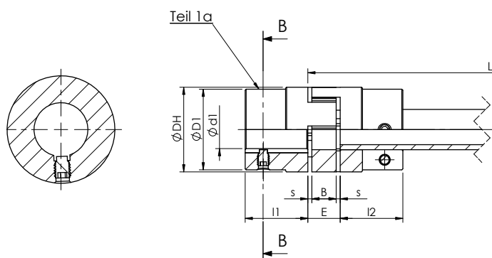
SCHNITT B-B
