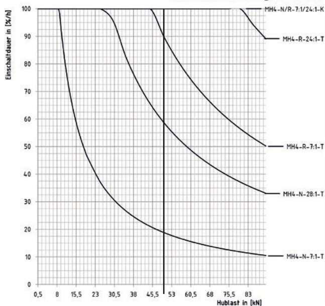
Einschaltdauerdiagramm MH4
