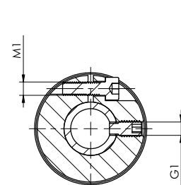
SCHNITT A-A
